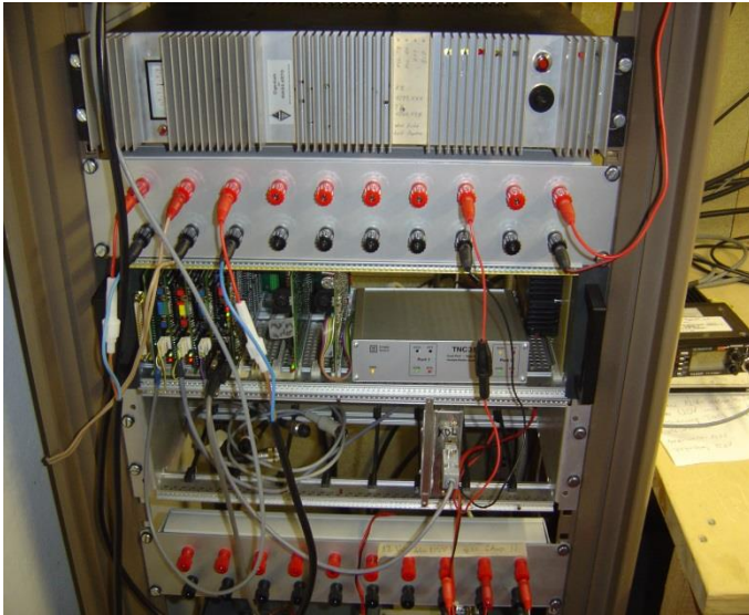
Einige Fotos der Anlagen von HB9EAS
